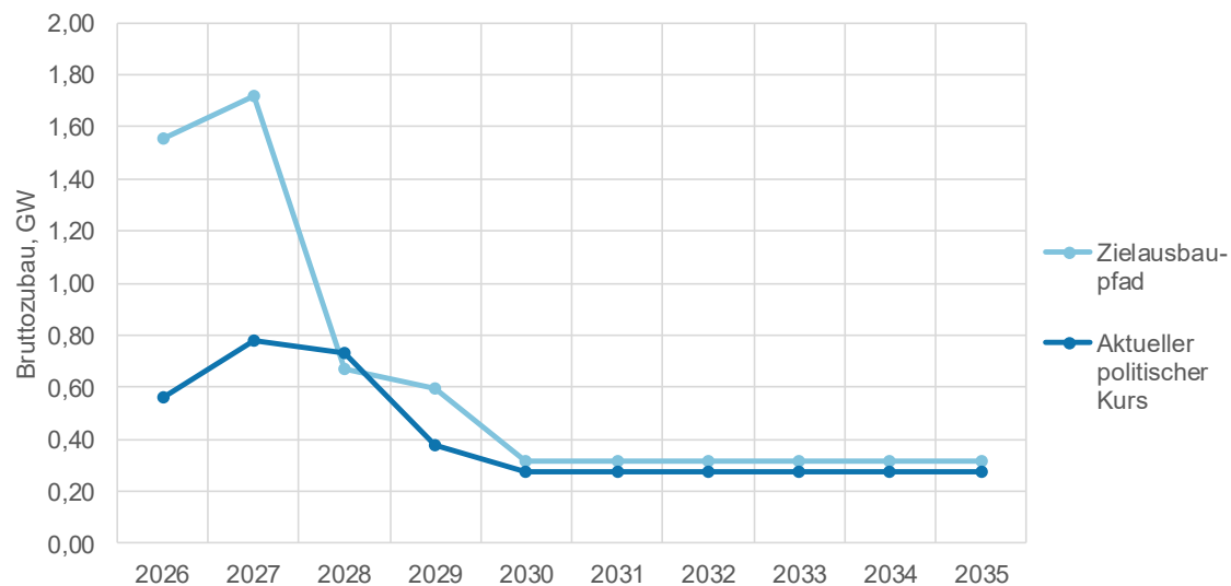
Abbildung 13: Szenariovergleich in GW – Biomasse (Biogas und Biomasse-HKW)
