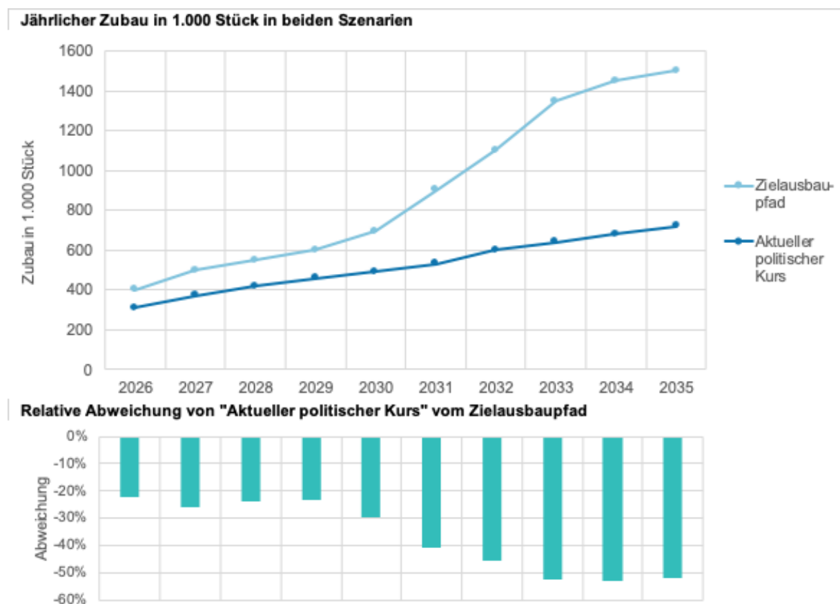
Abbildung 18: Szenarien Ausbaupfad und Aktueller politischer Kurs im Vergleich – Wärmepumpen
