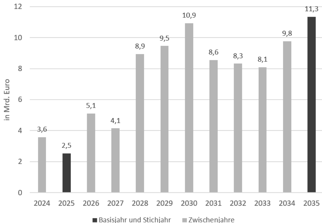
Abbildung 11: Investitionen in Windenergie-auf-See-Anlagen im Szenario Ausbauzielpfad bis 2035
